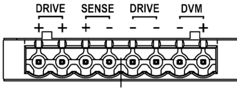
图 3-3 后背板端子
