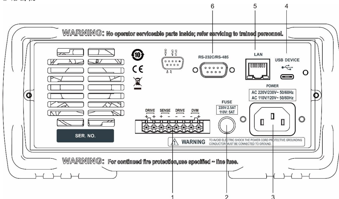
图 3-2 后面板
