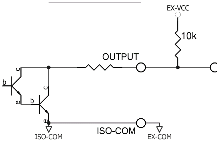
图 10-10 负逻辑输出
